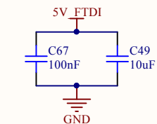
Filtrage alimentation FTDI
